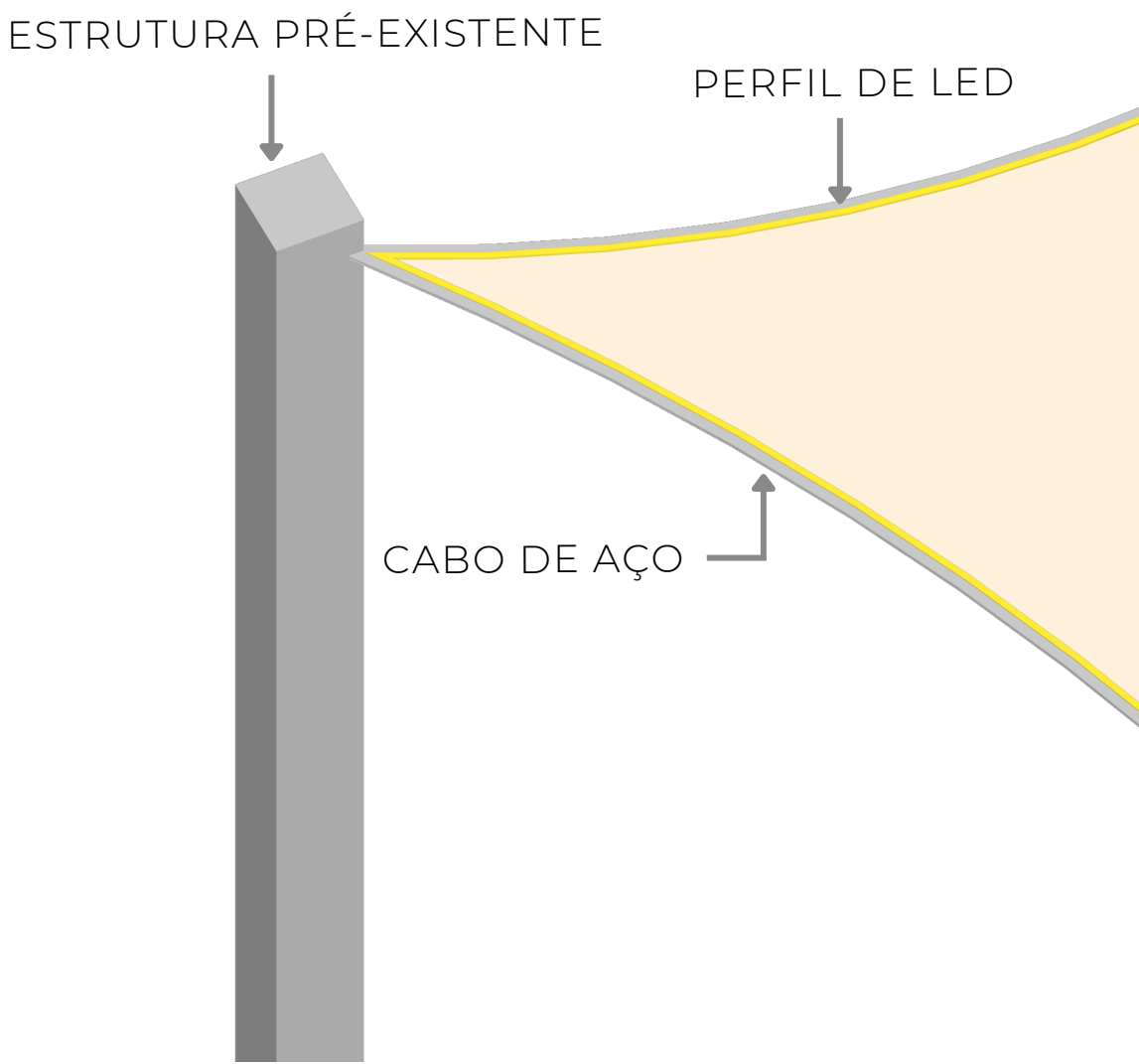
TECIDO TENSIONADO PROTEÇÃO E SOMBREAMENTO
